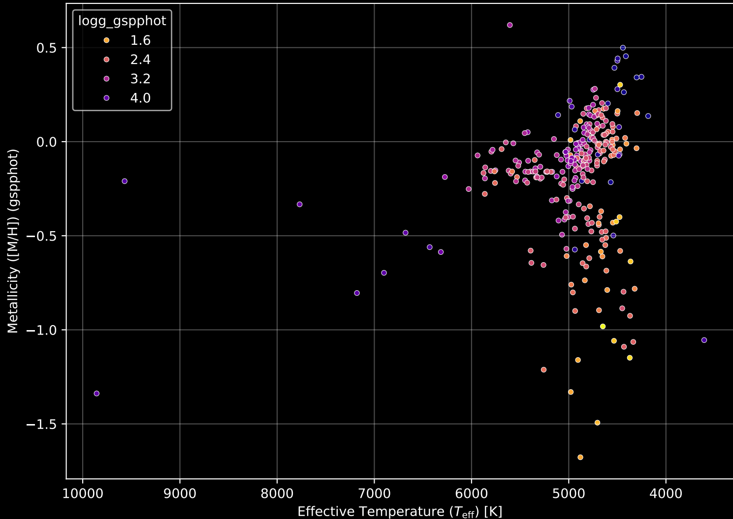
APOGEE DR17 Field: [345+14] Stellar Population Parameters (n= 302)
